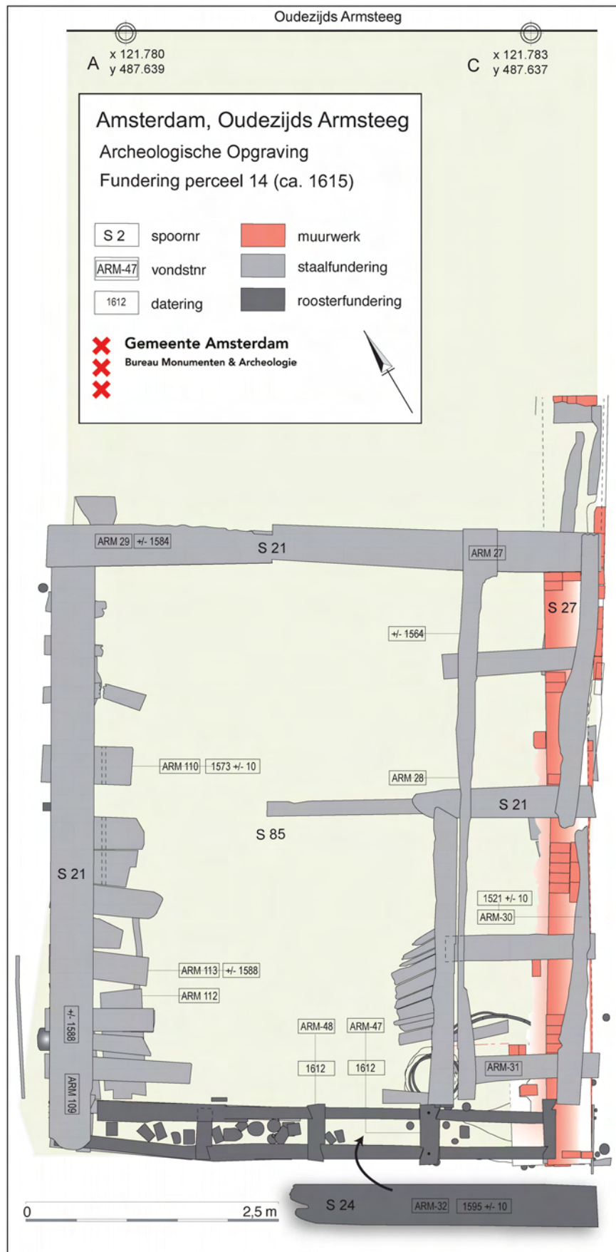
19 Grondplan van de verschillende funderingen (S 21) van Oudezijds Armsteeg 14, zonder de bakstenen muur S 2/ S 4
