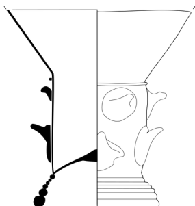
Schaal 1:2
