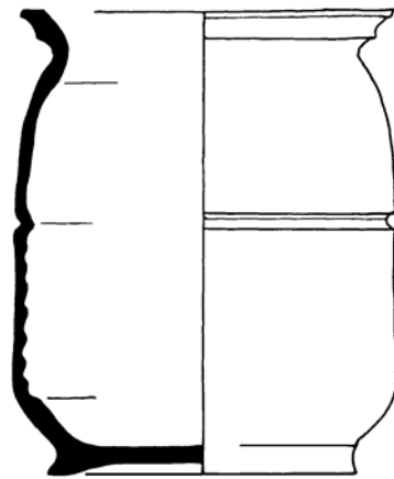
schaal 1:2
