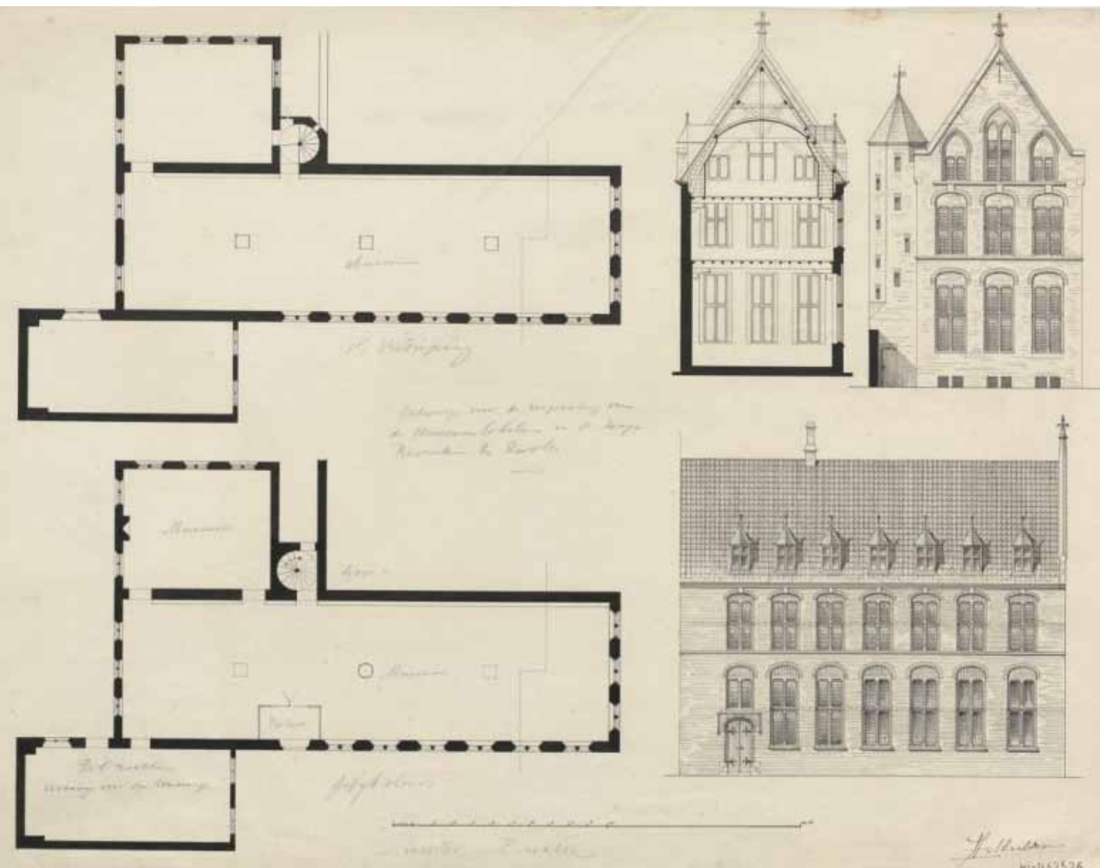
Refter van het Bethlehemklooster getekend in opdracht van de Rijksadviseurs in 1876.
