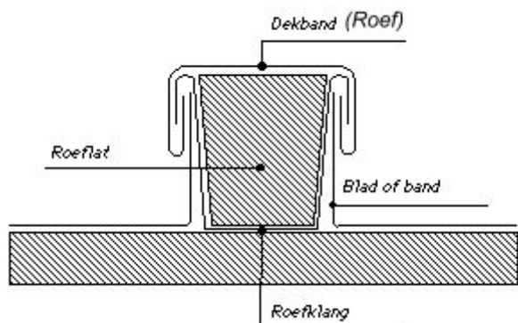
Detailtekening roevendak Botermarkt.
