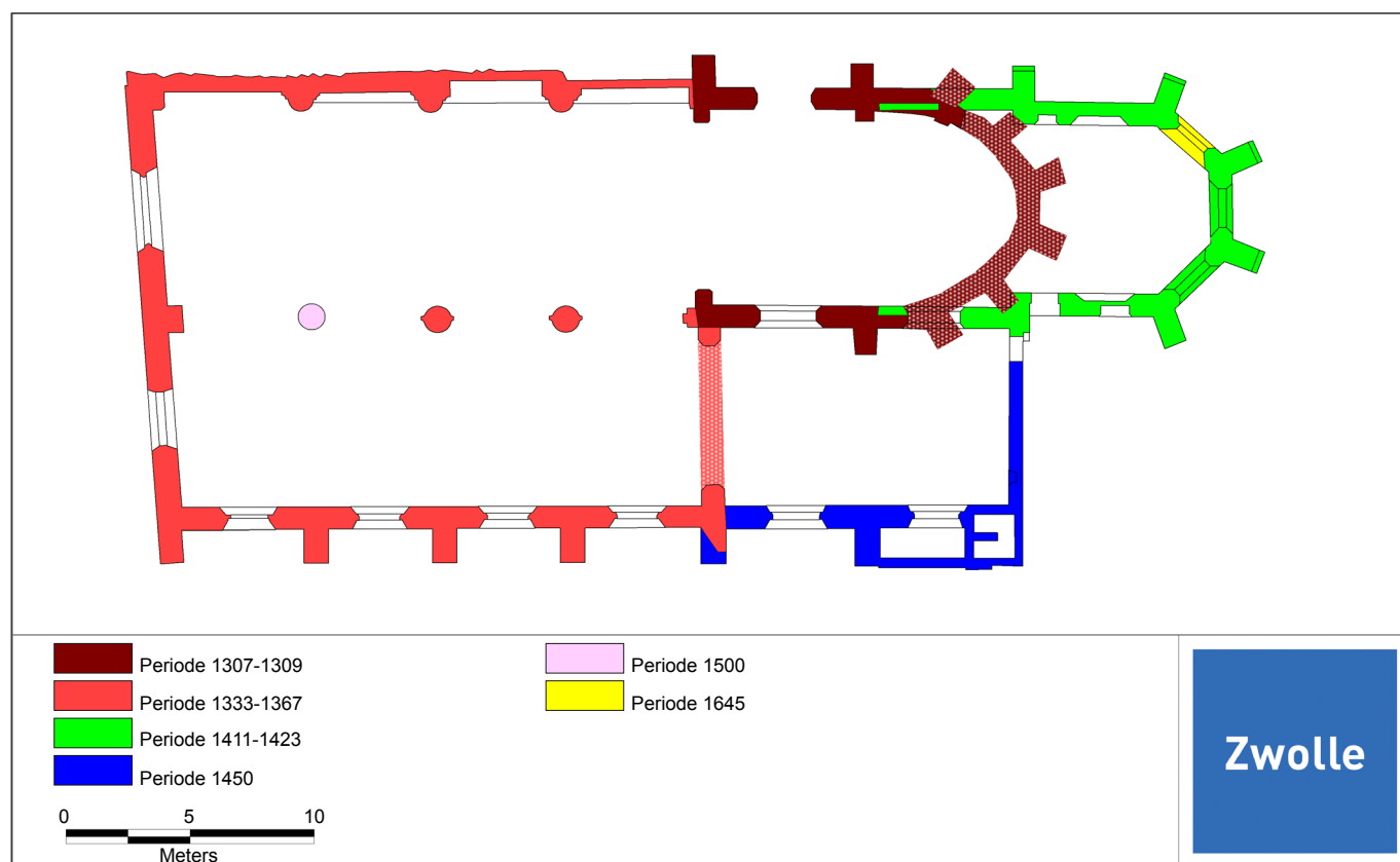
Plattegrond kerk met bouwperioden.
