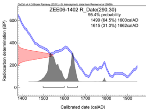
Afb. 1 Gekalibreerde resultaten van de datering.
