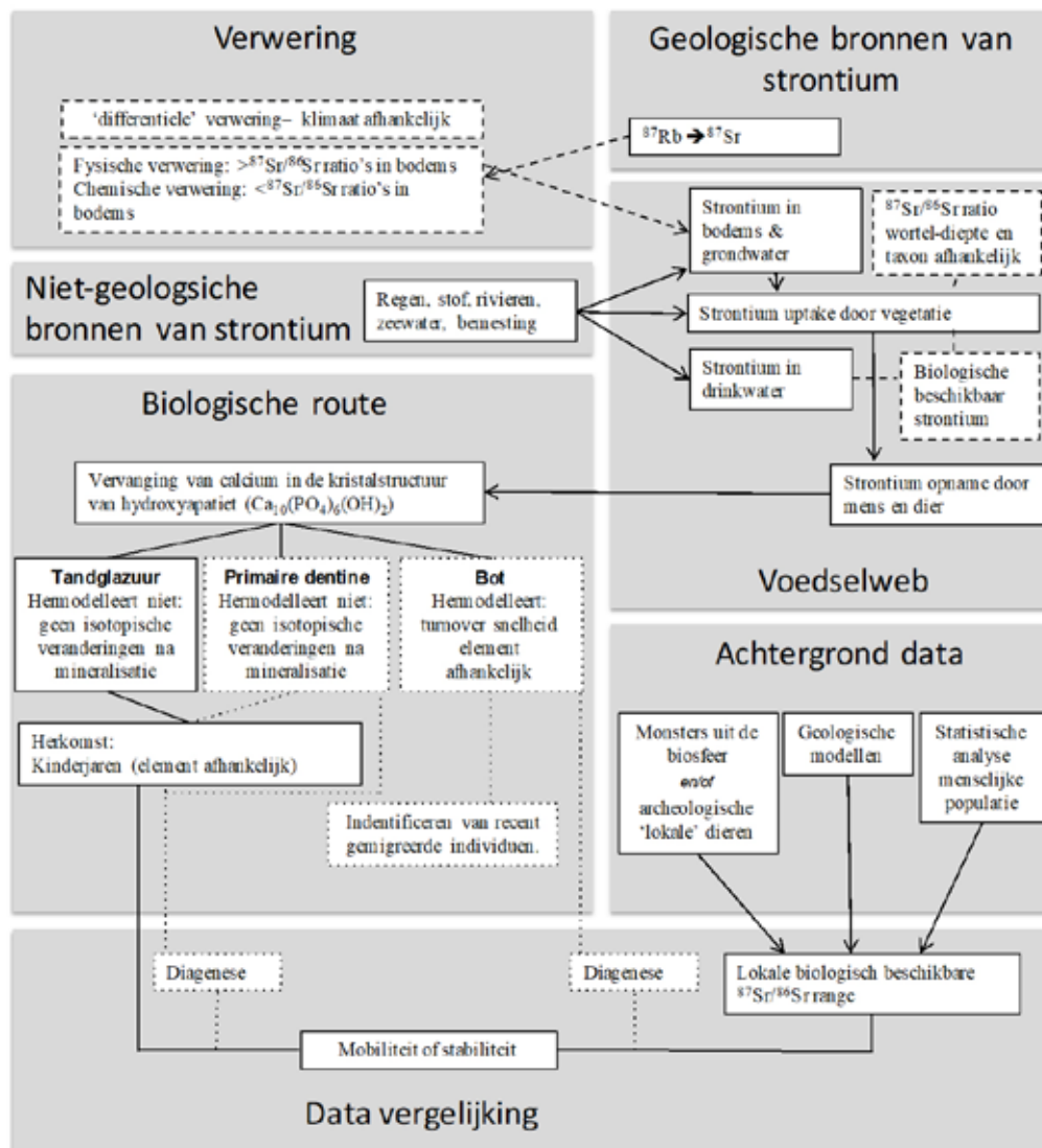
Schematische weergave van het principe van strontiumisotopenonderzoek.
