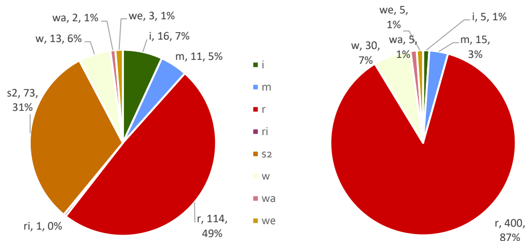
48 NF-86, bakselverhoudingen naar aantal scherven (N, links) en EVE (rechts)
