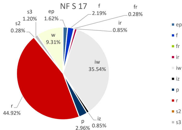
75 Afvalkuil S 5, bakselverhoudingen naar EVE
