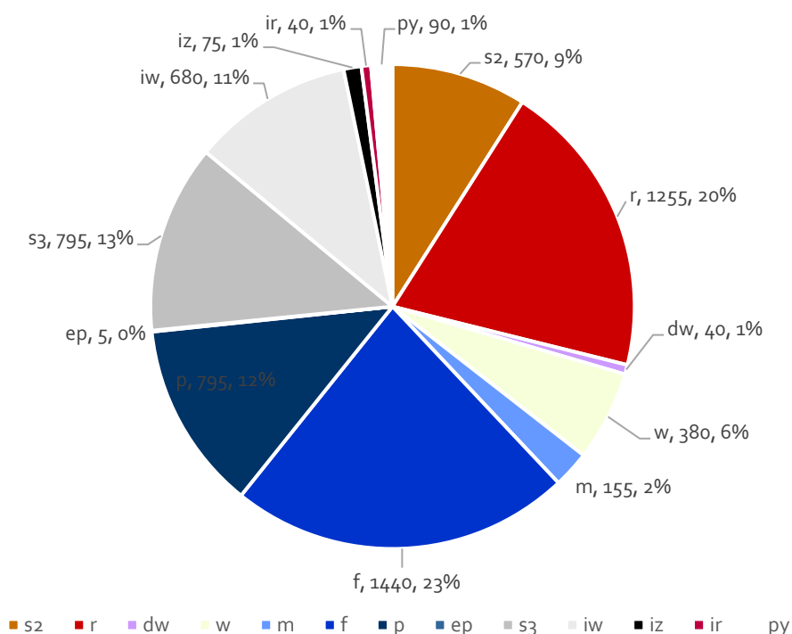
57 Foeliedwardsstraat 36, beerput S 17: bakselverhoudingen naar EVE
