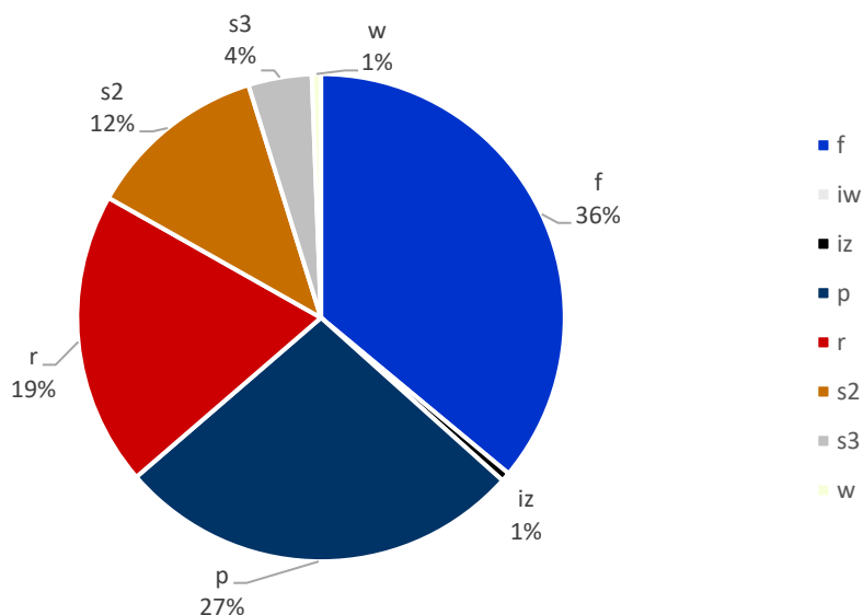
51 Beerput S 112, bakselverhoudingen naar EVE
